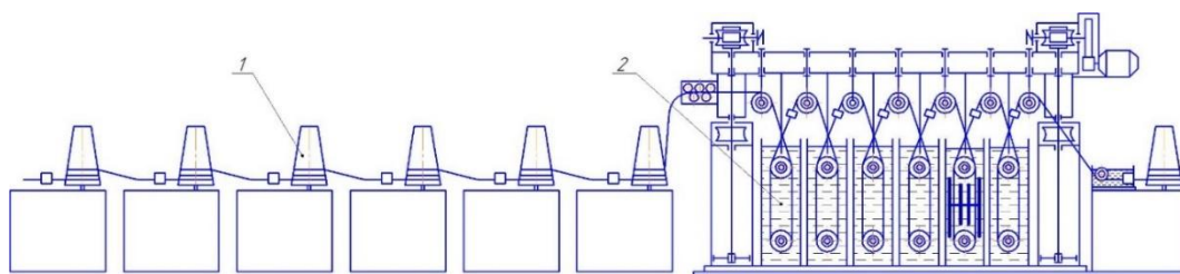
1 – тянущий барабан; 2 – установка латунирования
