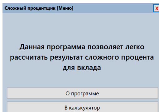
Рисунок 1 - Меню программы
