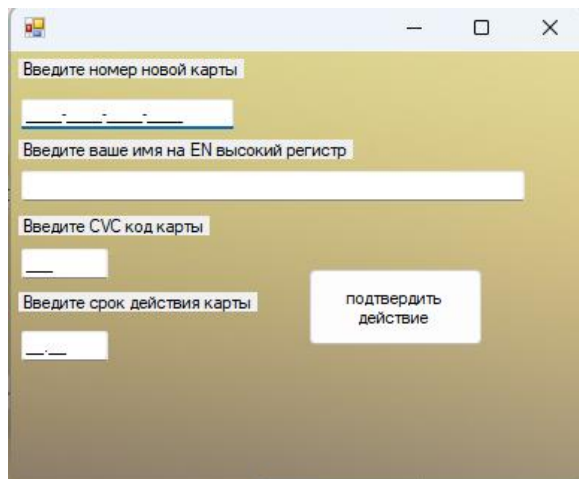
Рисунок 2 – добавление карты
